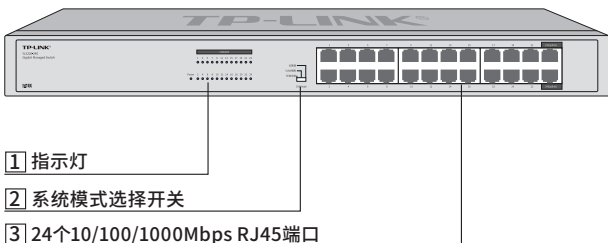
图1-2 前面板示意
